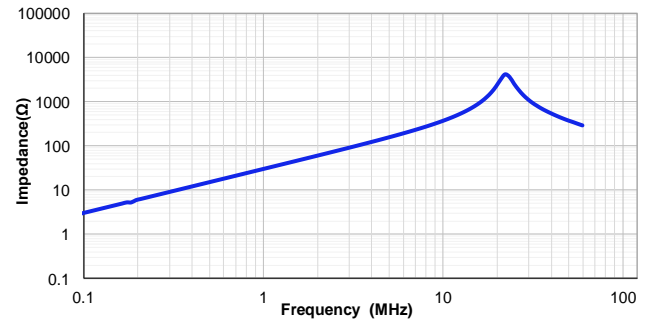
CSEB0530H-4R7M
