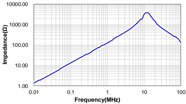
CPCF2920AS-470M
