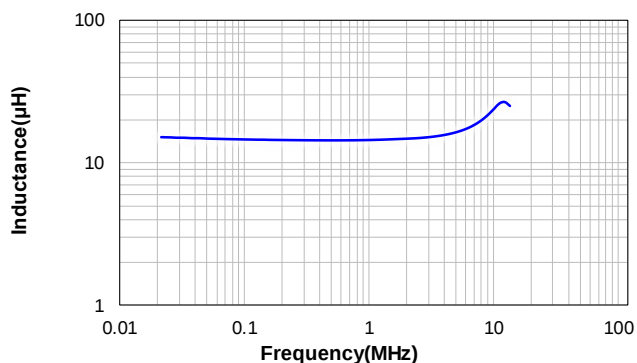
VSRU2420-200K
