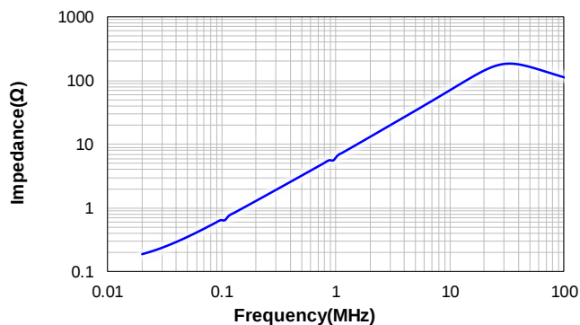
VSRU2415-2R2K
