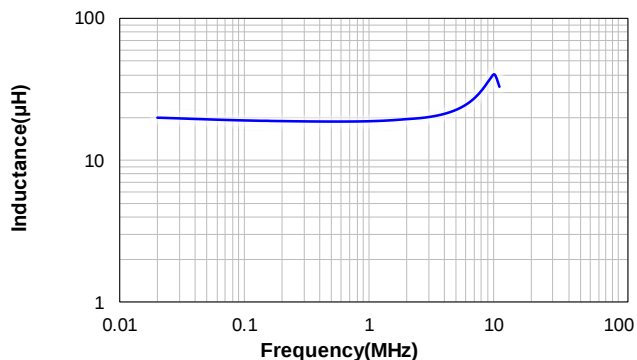
VSRU2420-200K
