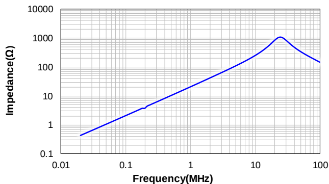
VSRU2415-3R3K
