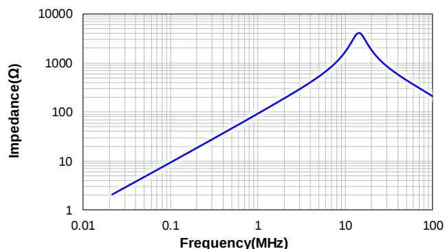
VSRU2420-200K
