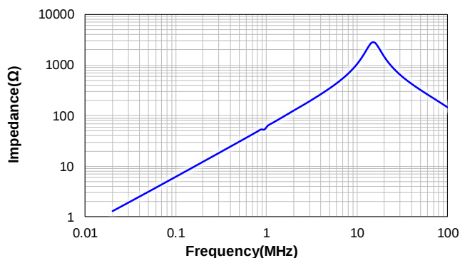
VSRU2420-300K
