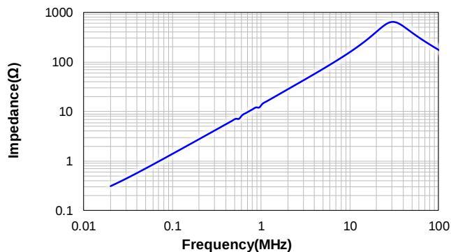
VSRU2415-2R2K
