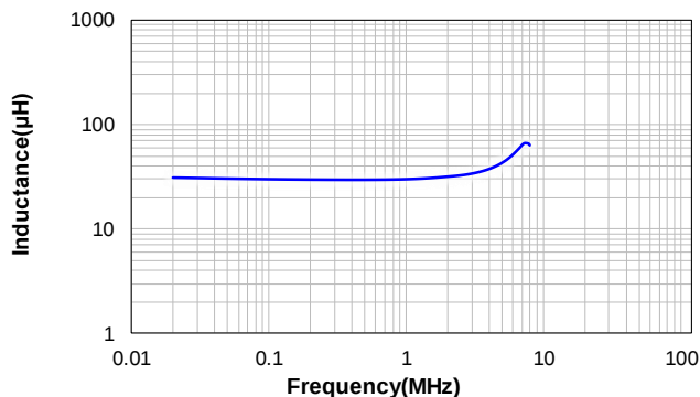
VSRU2420-300K
