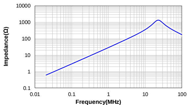
VSRU2417-150K
