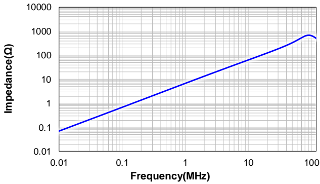
VSBX1275-2R8M
