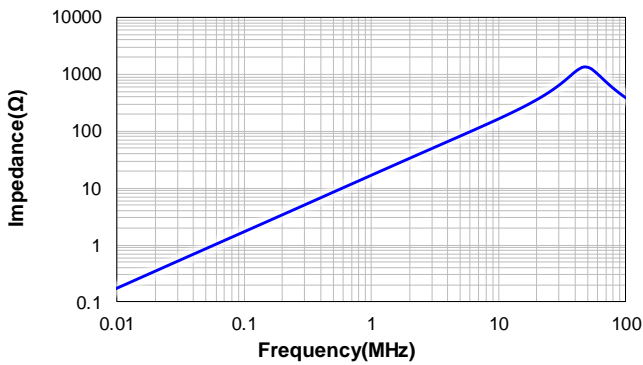
VSBX1275-5R2M
