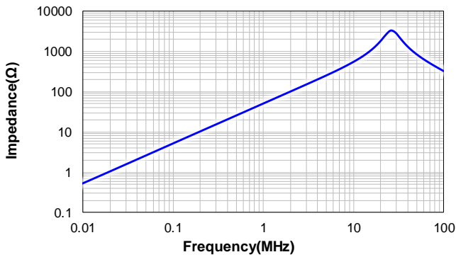
VSBX1275-8R4M
