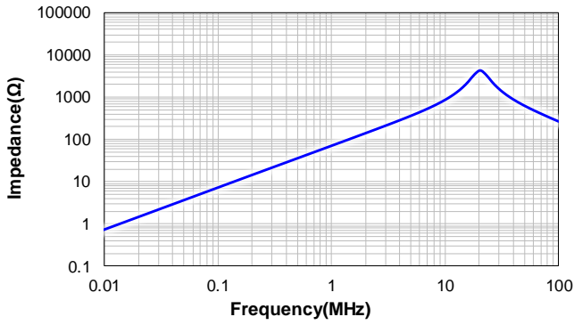
VSBX1275-220M
