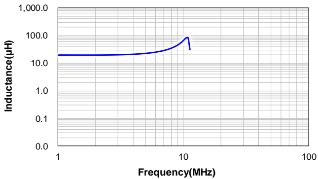
CSUC1210-200M:200M
