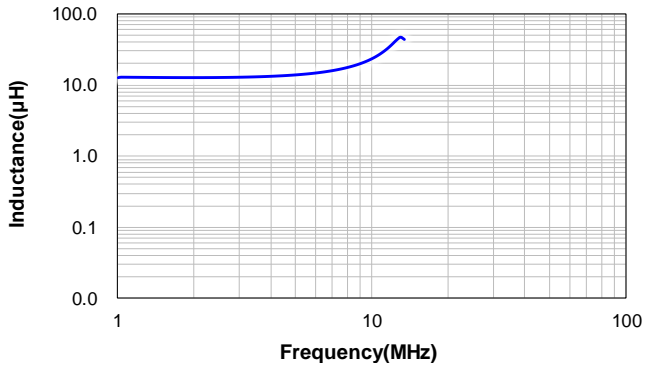
CSUC1210-200M:200M
