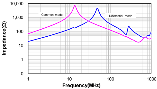
CSUC1210-200M:200M
