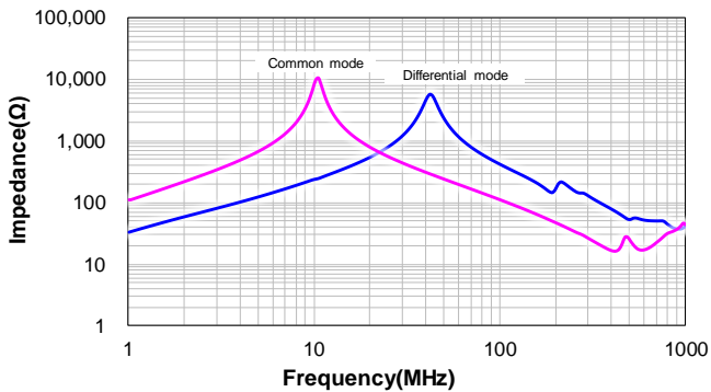
CSUC1210-200M:200M
