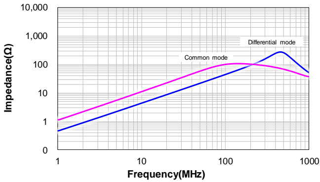
CSUC1208-1R0N:1R0N
