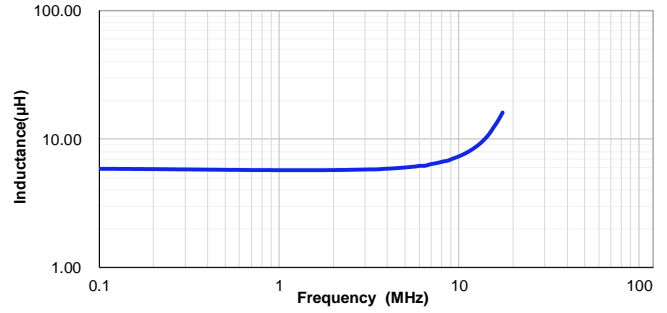
CSEB0730-5R6M
