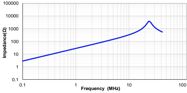
CSEB0730-4R7M
