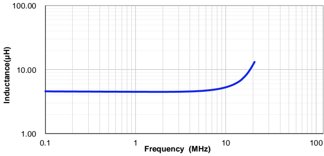
CSEB0730-4R7M
