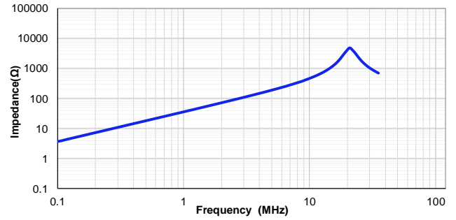
CSEB0730-5R6M
