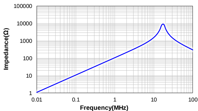
CSBA0860-180M
