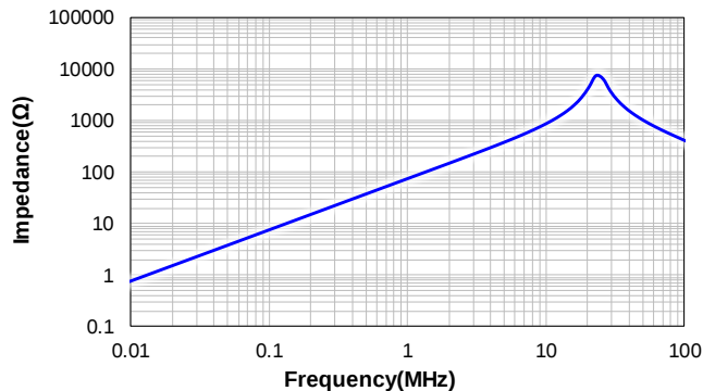
CSBA0860-120M
