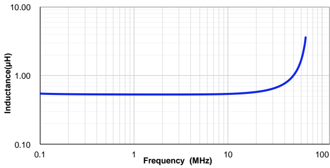
CSAB128050-R56M
