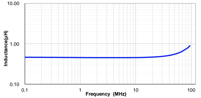
CSAB128050-R47M
