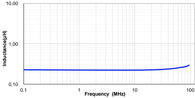
CSAB128050-R22M
